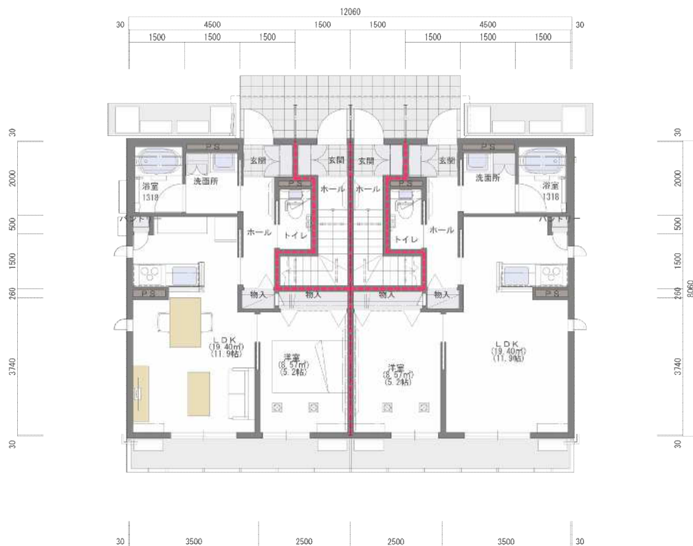
1階平面図 1/100
