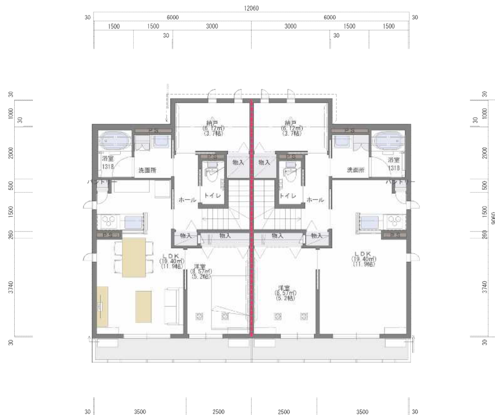
2階平面図 1/100
