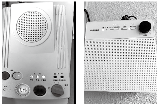
▲ IP 告知端末
